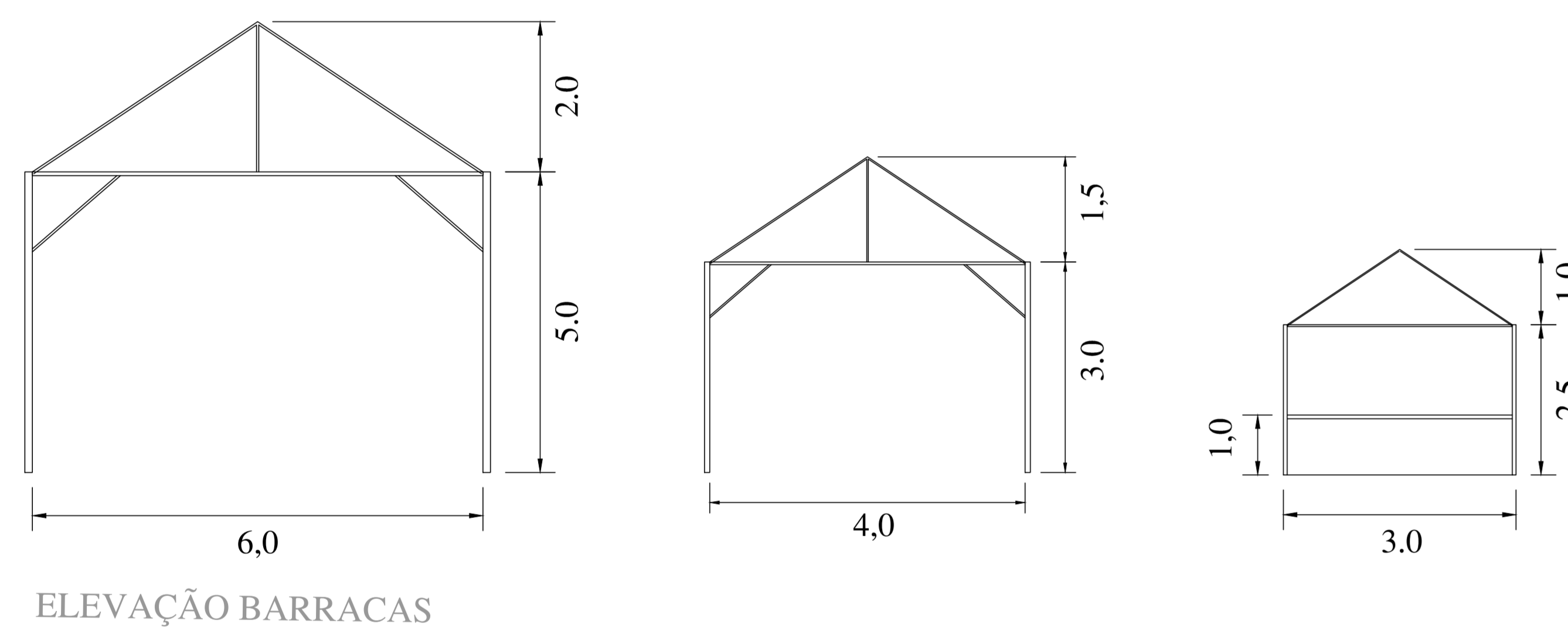
ELEVAÇÃO BARRACAS
