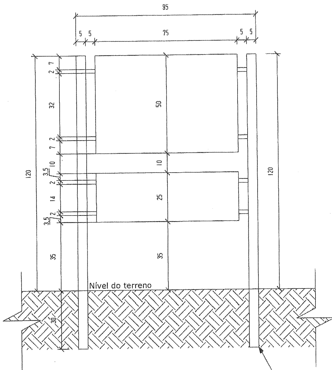
ELEVAÇÃO FRONTAL Escala - 1:100 Medidas em cm
